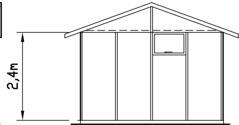
RIGHT ELEVATION
